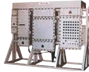
耐圧防爆形操作盤 Control Panel
